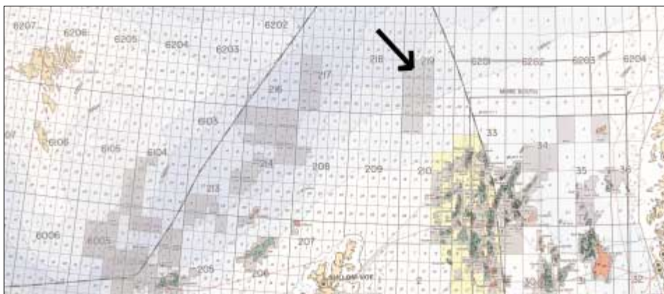
Vit sjggja á kortinum kendu olju- og gassfeltini í bretsrum og norskrum øki. Pílin sýsir Ben Nevis struktúrinn har norðuri í bretsrum øki miðskeiðis millum føroyska og norska markið.
