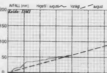
Avfallið 0,1 mm - mált frá 20.08. kl 06 00 -21.08. kl 06 00 . Avfallið higartil í august: 55,8 mm
