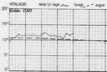
Hitalagið mált frá 20.08. kl 06 00 -21.08. kl 06 00 . Hitin í gjár: 12,2°C. Mest hiti máldur í aug. 22,0°
