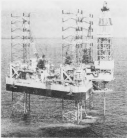
A myndin sýgja vit ein av boripallunum - sum eru nógv bruktir í Norðsjónum - Maersk hevur borað nógva staðni kring heimin. Fær Maersk arbeiðið í Lopra, verður tað fyrstu ferð, at teir bora á landi í Evropa.
